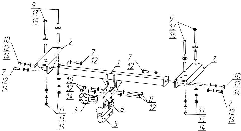
Схема монтажа
