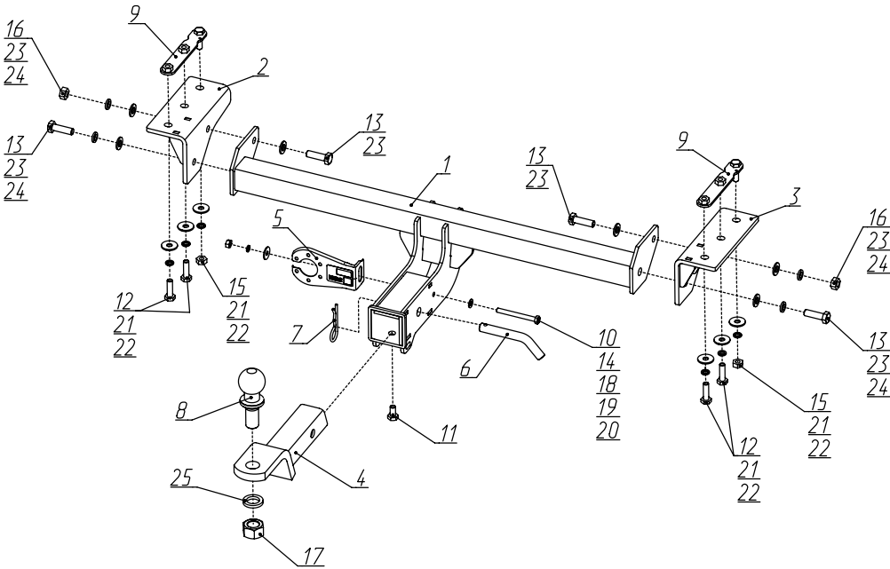
Схема монтажа
